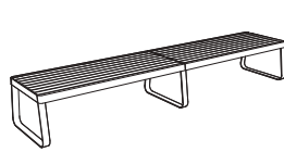
I1-621 3000 × 652 × 457
