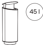
U20-1411 363 × 363 × 984
