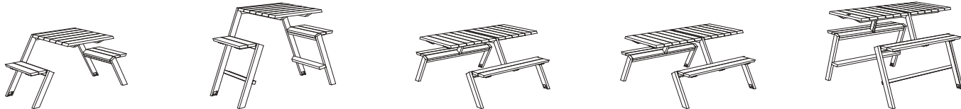
U6-121 1630 × 810 × 780 U6-171 1630 × 810 × 1100 U6-221 1576 × 1630 × 780 U6-222 1576 × 1630 × 780 U6-271 1576 × 1630 × 1100
