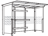
X1-S310-SS 4170 × 1738 × 2605
