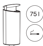
U20-5420 423 × 423 × 1090
