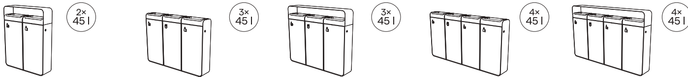
I20-2411 864 × 233 × 1094 I20-3401 1294 × 233 × 947 I20-3411 1294 × 233 × 1094 I20-4401 1724 × 233 × 947 I20-4411 1724 × 233 × 1094
