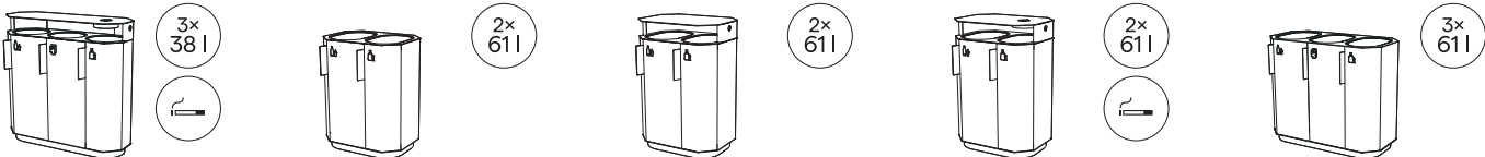
A20-3221 974 × 348 × 953 A20-7201 656 × 477 × 827 A20-7211 660 × 481 × 953 A20-7221 660 × 481 × 953 A20-8201 970 × 510 × 827
