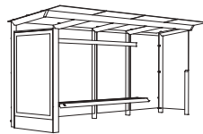
X1-430-SS+CLV 5630 × 1738 × 2605
