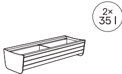
I30-500E 1374 × 510 × 300
